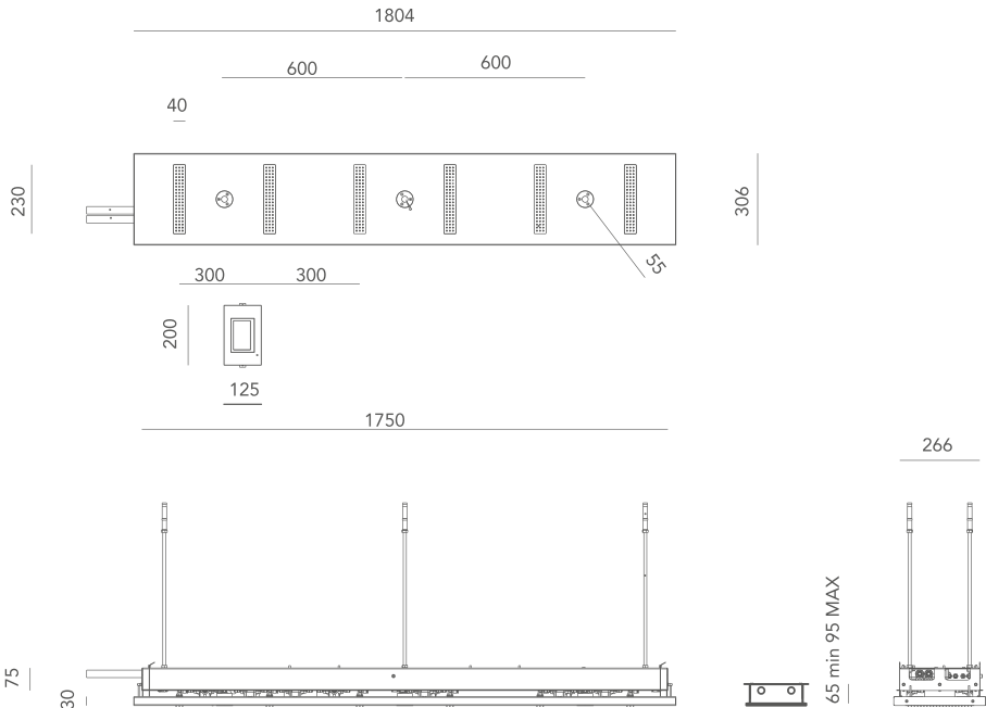
Spessore parete controsoffitto da 5 a 40mm
