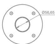
Recessed Mini Projector Niche
