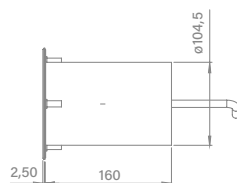
Recessed Mini Projector
